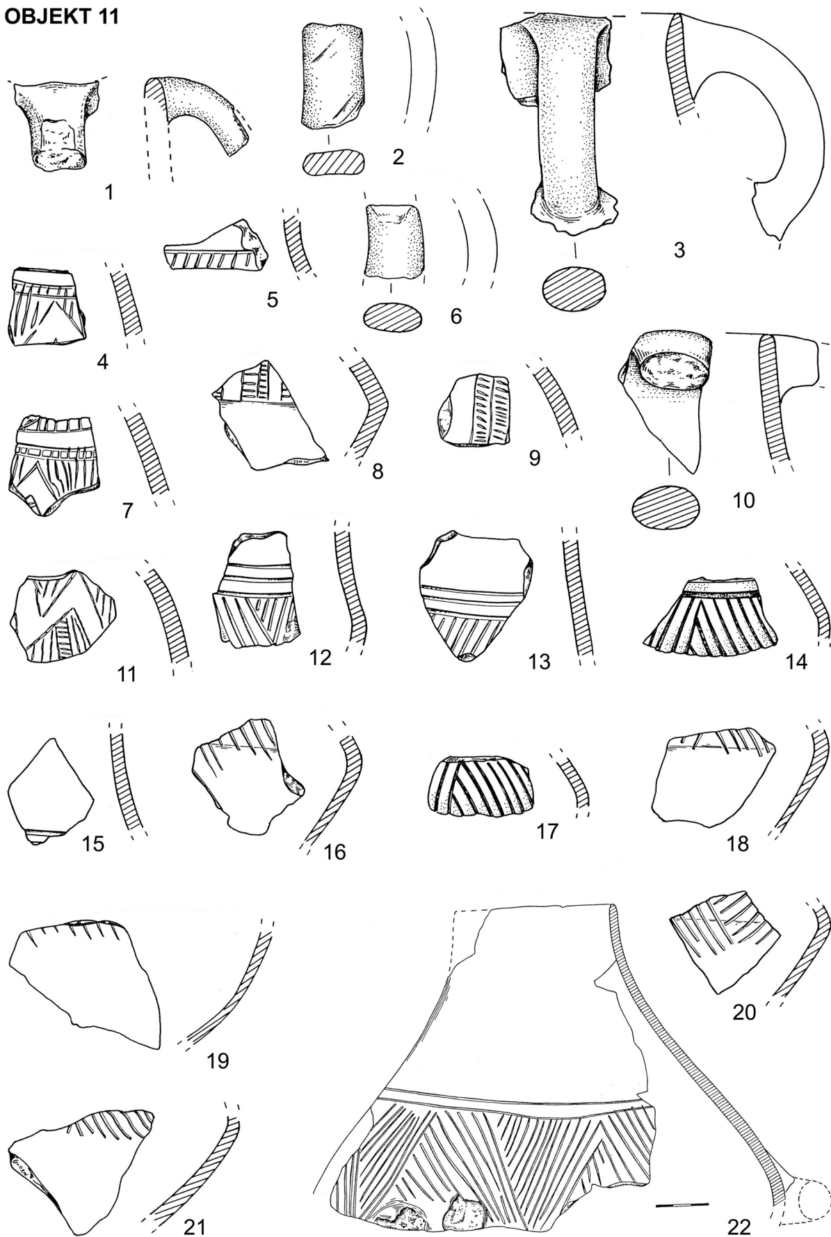
Obr. 18. Praha-Ďáblice. Keramika z objektu 11. Měřítka 2:3, předmět s grafickým měřítkem 1:3. Kreslila M. Fábiková
